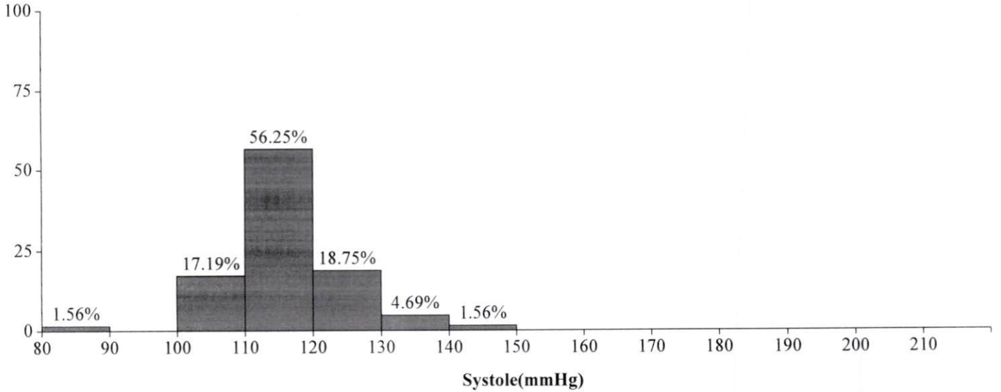
Histogramme(Tout)
